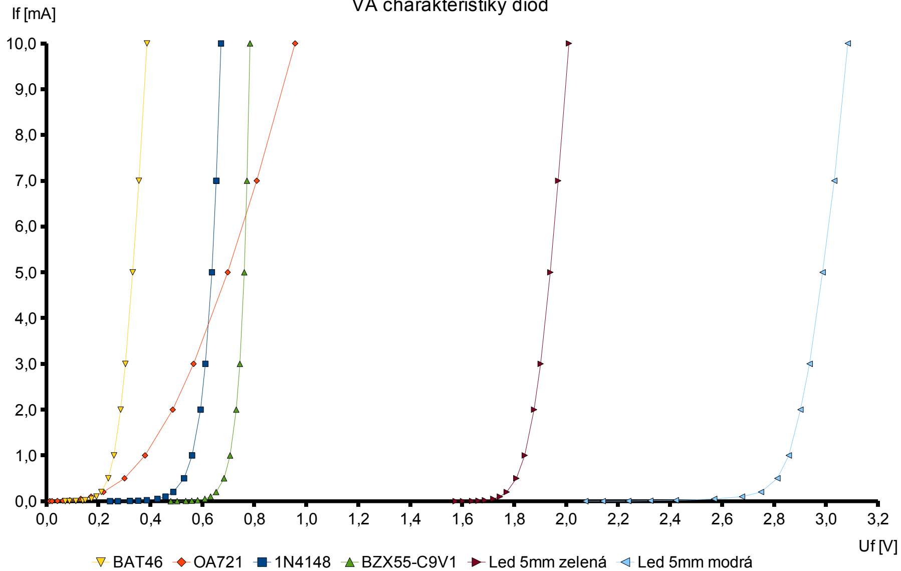
VA charakteristiky diod
